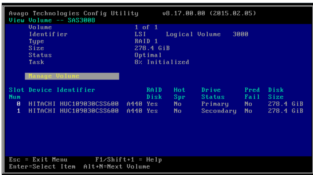
图 3-36 RAID 阵列界面
